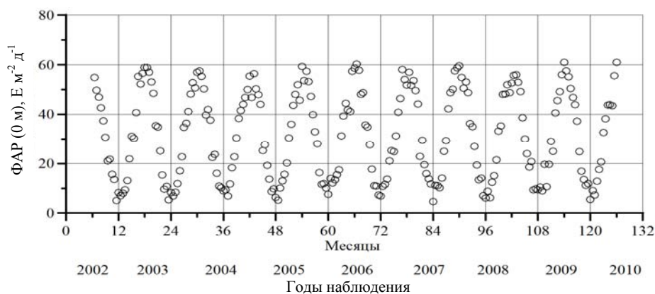
Рис. 2. Изменение падающей на поверхность моря фотосинтетически активной радиации (ФАР) в западной глубоководной части Черного моря (по данным сканера цвета MODIS).
