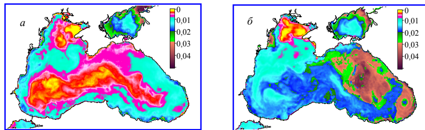
Рис. 7. Примеры пространственного распределения b_{bp}(555) ( \text{в м}^{-1} ) в акватории Черного моря: a – первая половина июня 2005 г.; b – первая половина июня 2012 г.
